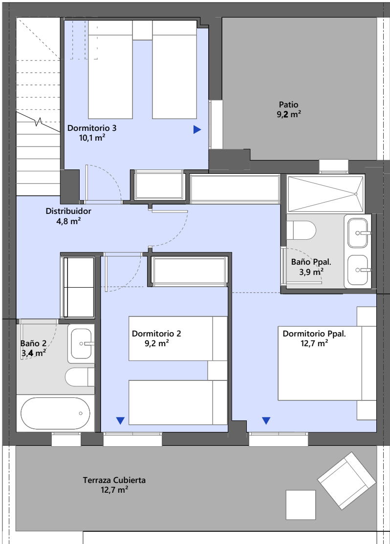
PLANTA SOTANO
