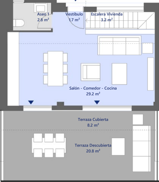
Planta primera
