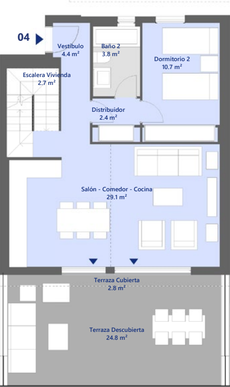
Planta baja
