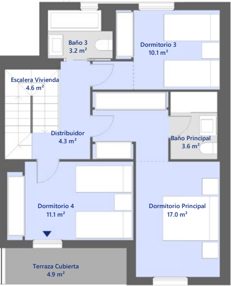
Planta primera
