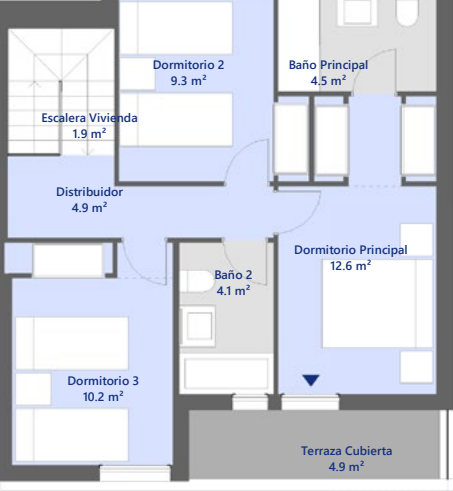
Planta primera
