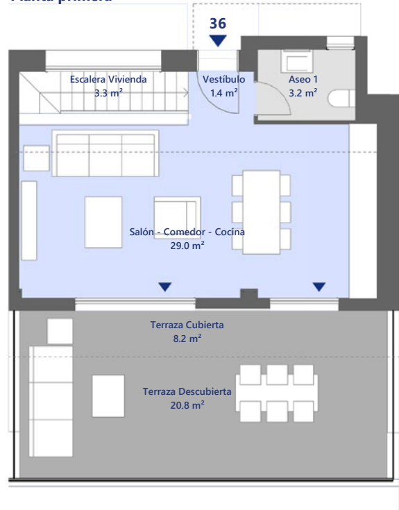
Planta primera
