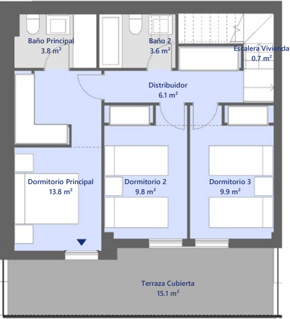
Planta baja
